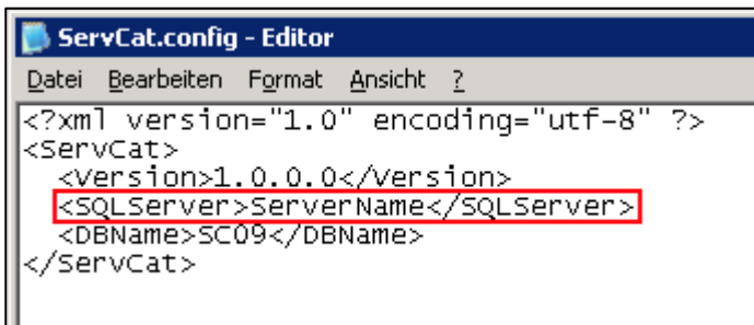
Abbildung 5: ServCat.config
